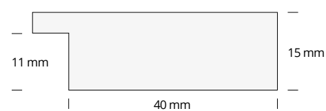
Sezione cornice dimensioni reali Frame section real sizes
